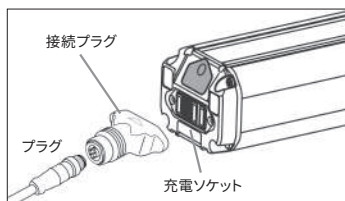
充電器のプラグと充電ソケットの間に接続プラグ(アダプター)を使用します
