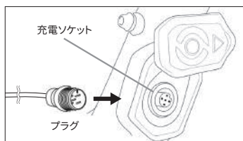
充電器のプラグを車体の充電ソケットに接続します
